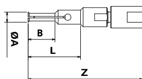
Expander MP50507 bis MP50811
