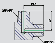
ADF302 Adapter Art.Nr. 7200207
