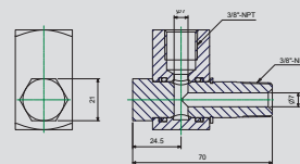
BG9705 Schwenkbare Kupplung für hohen Durchsatz Art.Nr. 79000661
