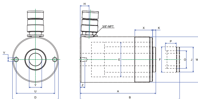
Zylinderbohrung
