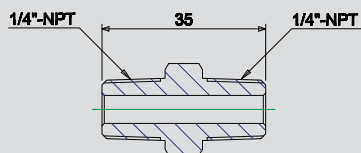
ADO303 Sechskantnippel Art.Nr. 7200218
