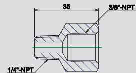
ADF304 Adapter Art.Nr. 7200209
