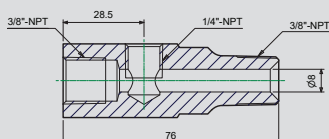
ADG323 T-Stück für Manometer High Flow Art.Nr. 7299232
