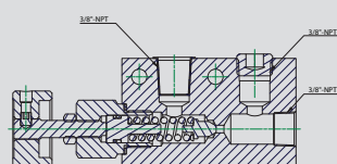
BG9623 Druckentlastungs- ventil Art.Nr. 7200227
