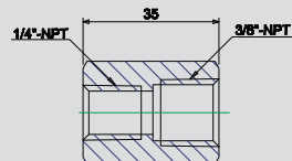
ADO203 Reduzierstück Art.Nr. 7200160
