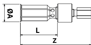
Expander MP51214 bis MP56576
