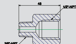
ADI303 Verbindungsstück Art.Nr. 7200212
