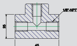
ADG303 T-Stück Art.Nr. 7200204
